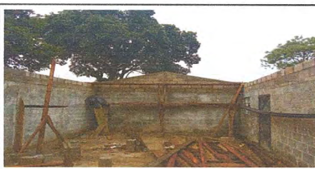
Foto 6: Elaboración de dos hiladas de block para subir la altura del aula módulo 3.
