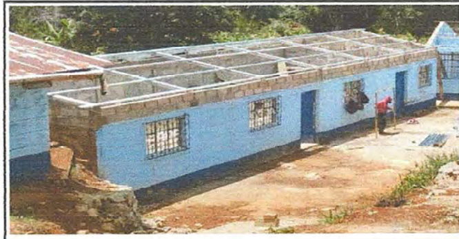
Foto 12: Instalación de estructuras módulo 3.
